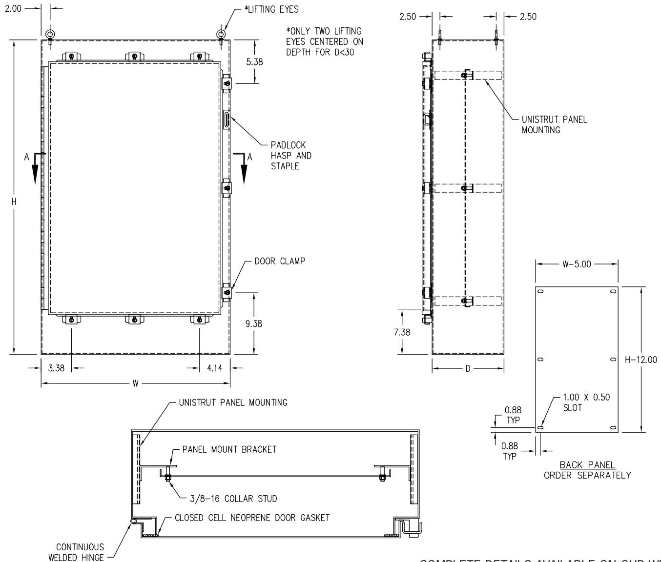
SECTION A-A
